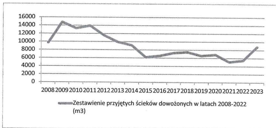
Wykres Nr 9. Ilość przyjętych ścieków dowożonych w latach 2008 - 2023r.
